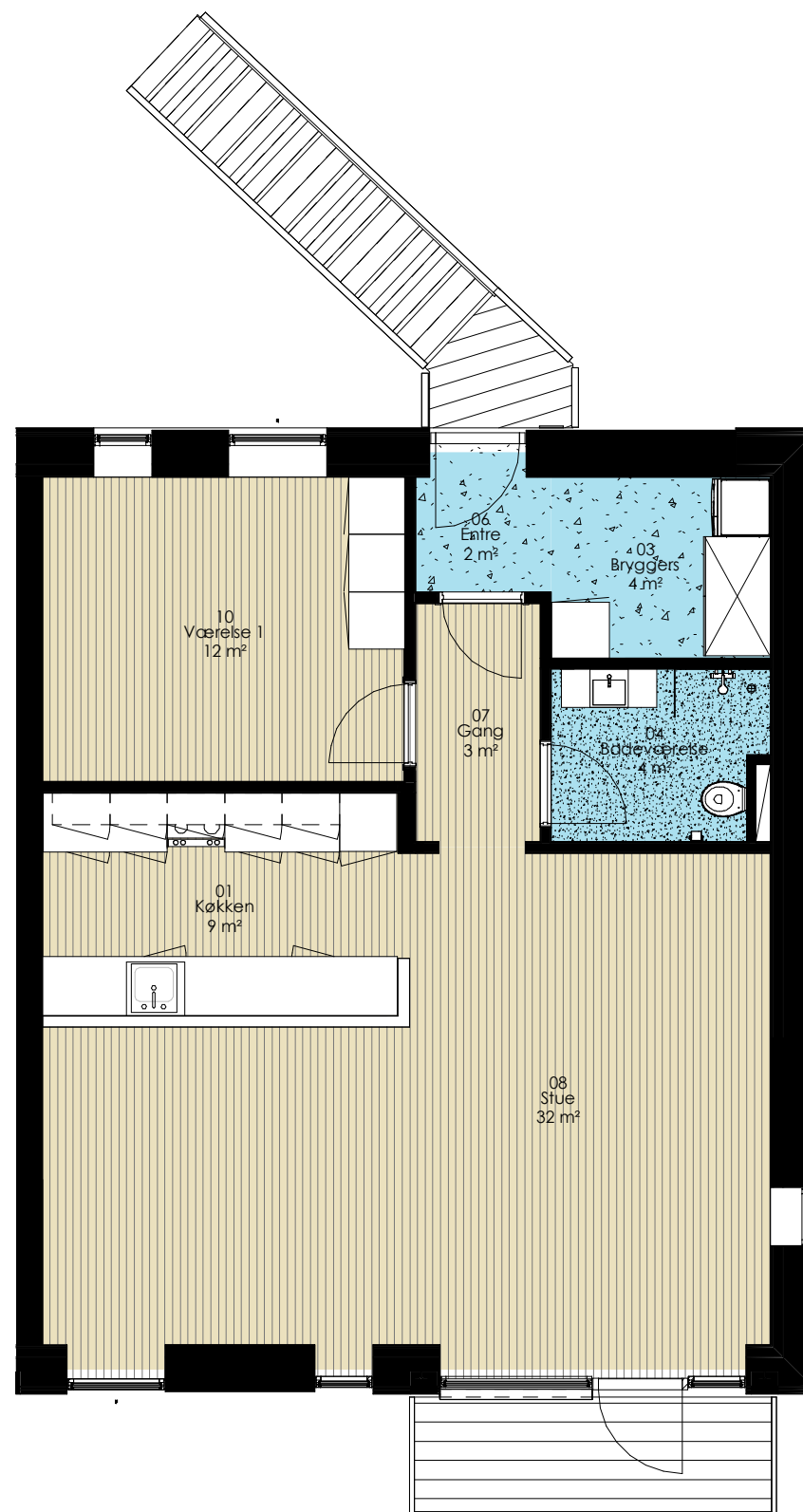
Lejl. 1B.1 - Type AB - 1.sal 1:75
