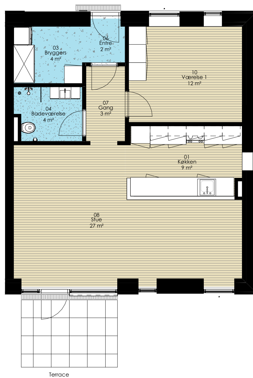
Lejl. 3A - Type AB 01 - stue 1:75
