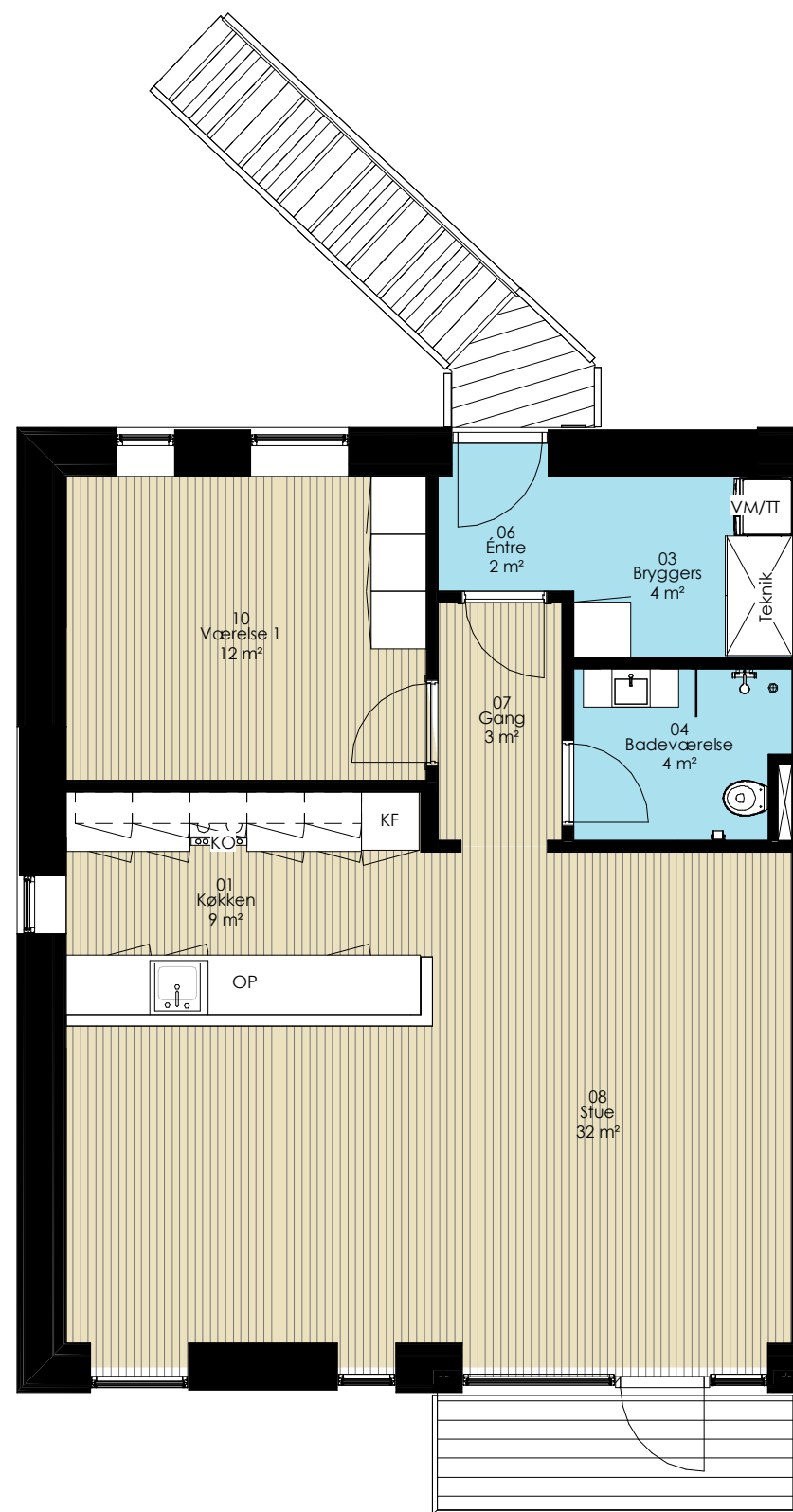
Lejl. 4A.1 - Type AB - 1.sal 1:75
