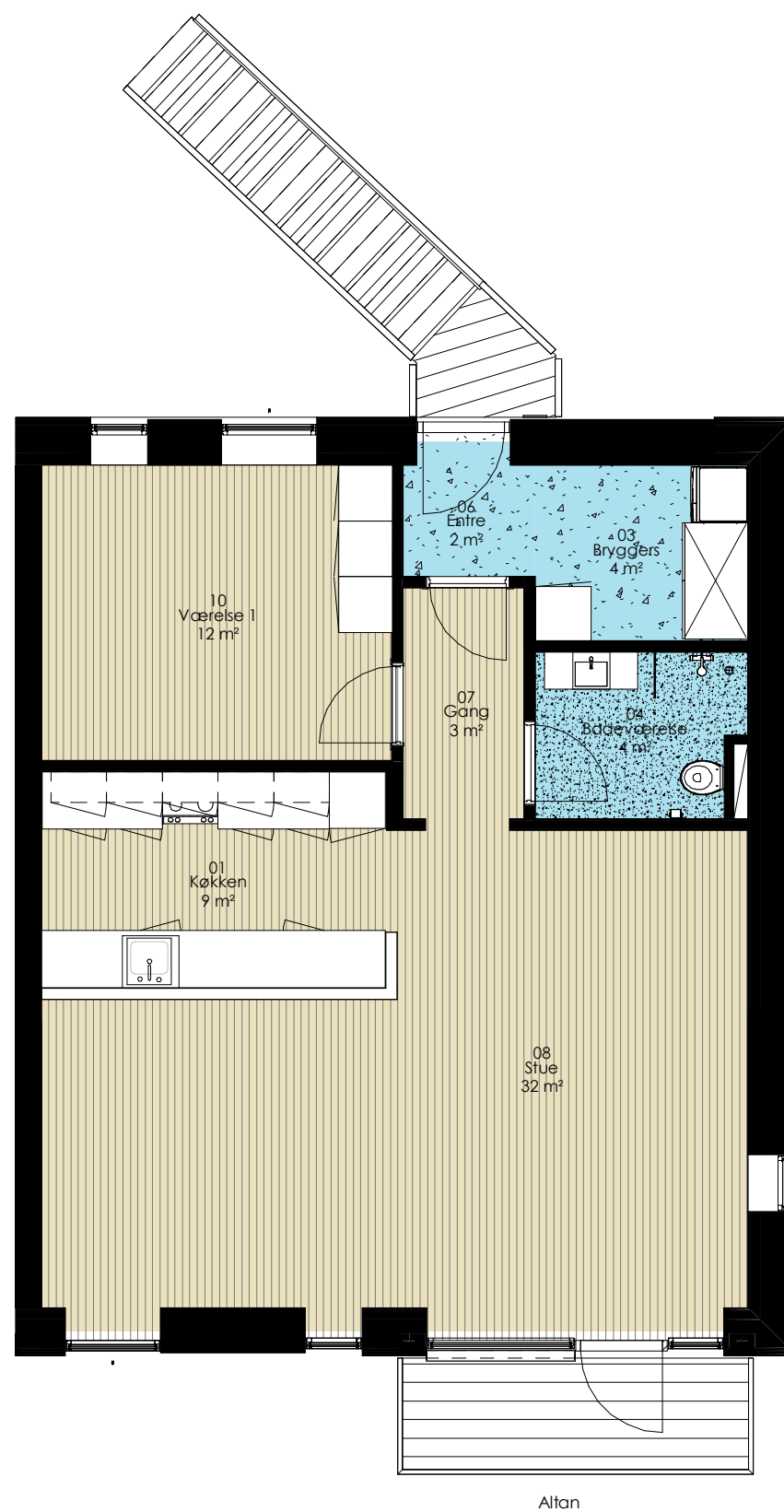
Lejl. 4C.1 - Type AB - 1.sal 1 : 75
