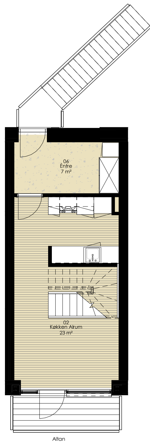
Lejl. 6B - Type CBA - 1.sal 1 : 75
