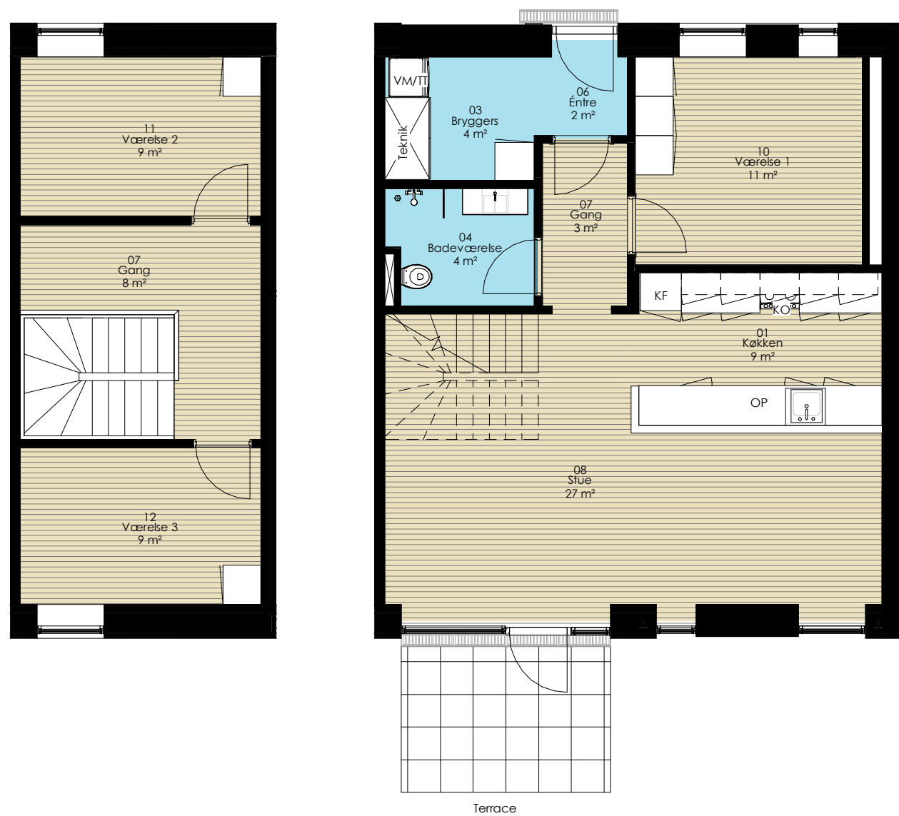
Lejl. 6C - Type ABC 02 - 1.sal 1:75
