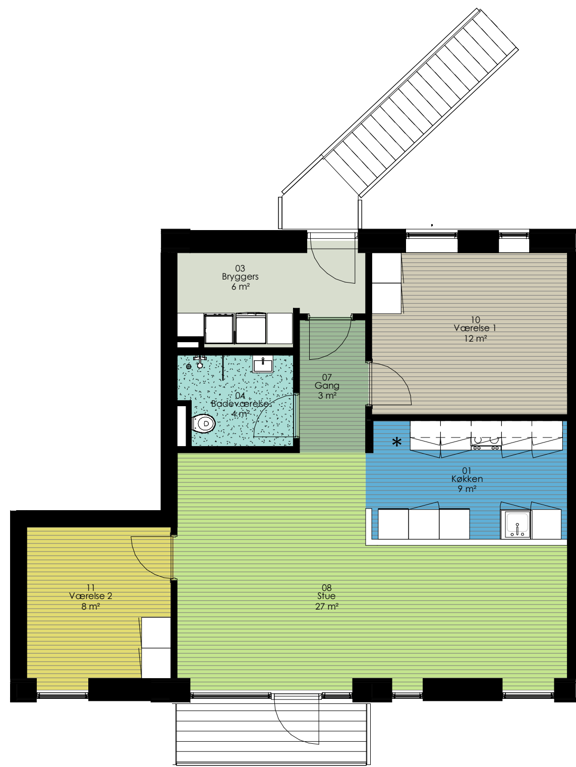
Lejl. 4L.1 - Type A2 1 : 75
